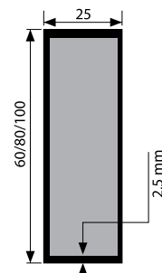
Holmquerschnitt Vangens snit Tverrsnitt vange 2,5 mm
